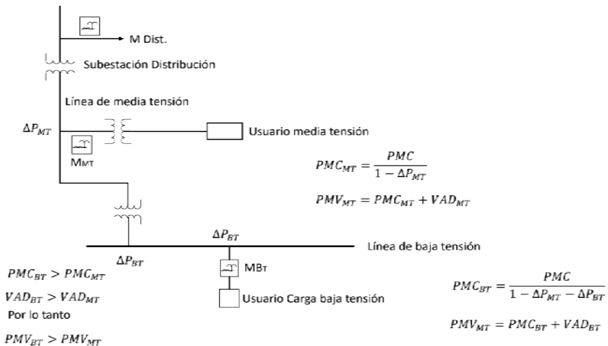
Figura 1. Diagrama unifilar sistema de transporte de energía en una empresa distribuidora
